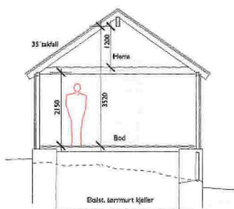
Omsøkt istandsetting, tverrsnitt
