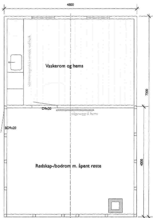
Omsøkt istandsetting, plantegning bodrom
