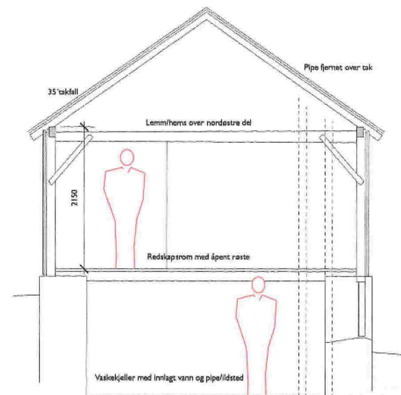
Eksisterende uthus, tverrsnitt. Se også fotodokumentasjon
