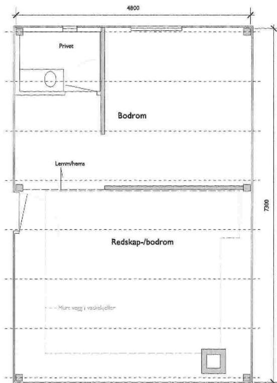
Eksisterende uthus, plantegning. Se også fotodokumentasjon
