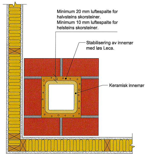
Leca Rehabiliteringssytem (luftet løsnng) i teglskorstein. Stabilisering av innerrør med løs Leca.
