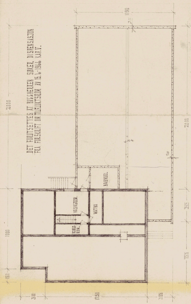
PLAN KJELLER OG FUNDAMENT
