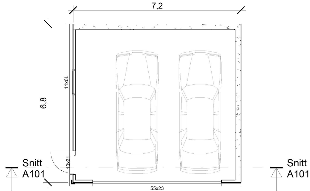
plan 1.etg 1 : 100
