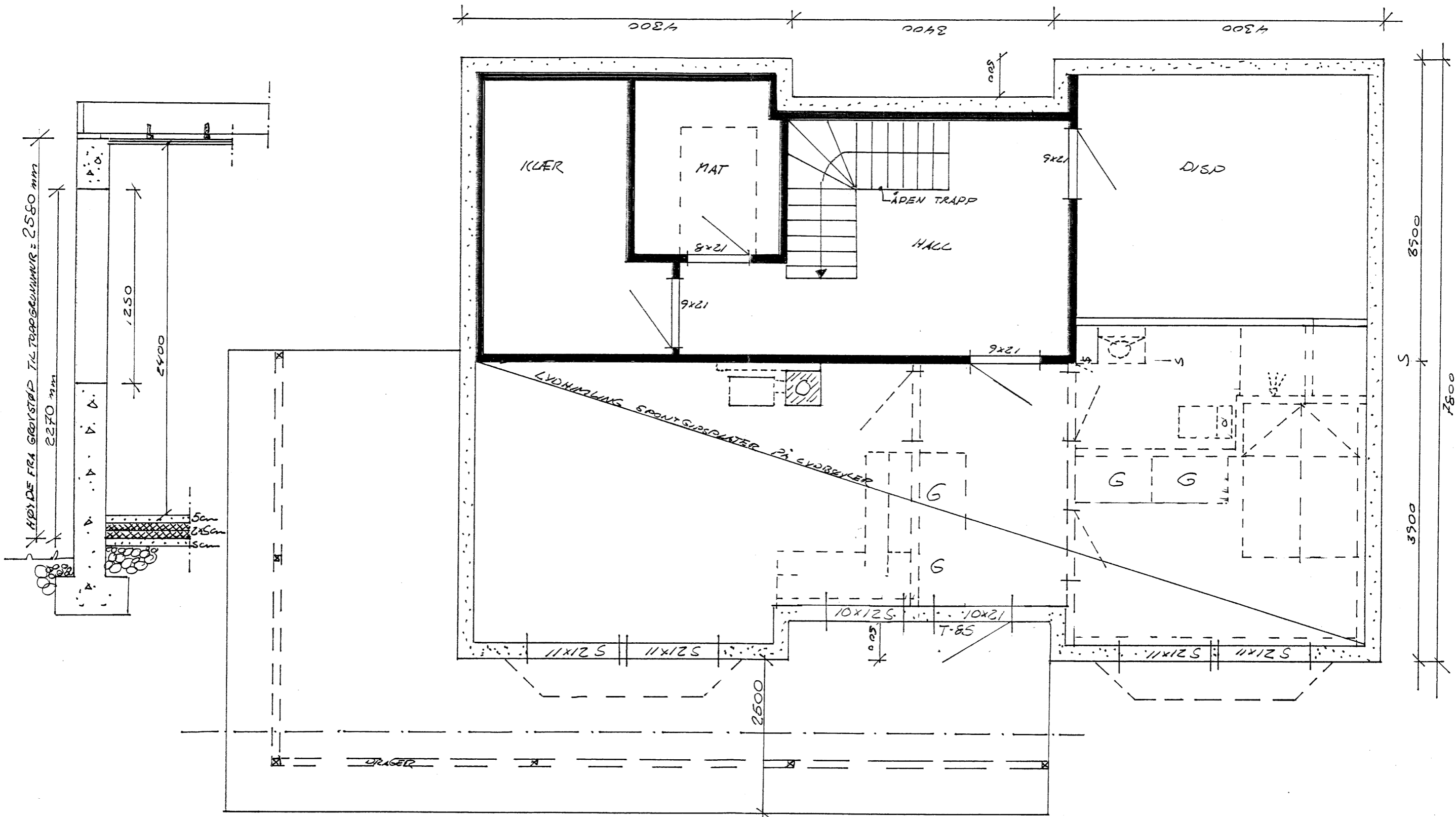
Kjellerplan for Rune Nordrik 1:50 16/5-97 GNR:21 BUR39,
