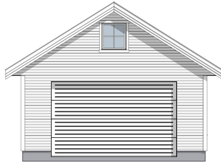
1:100 Fasad Nord
