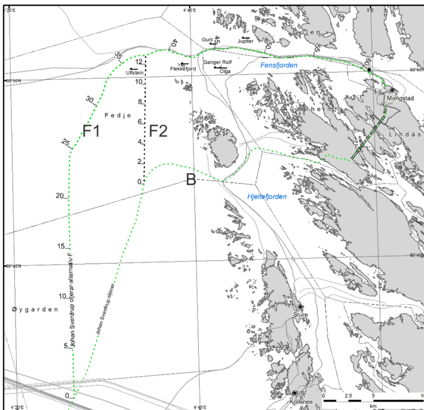
Figur 2: Kartet viser traséene (stiplet grønt) Statoil har vurdert for å frakte olje til Mongstad fra Johan Sverdrup feltet. Eit av alternativene var å krysse under Lurefjord-systemet med ein oljerørledning i tunell.
