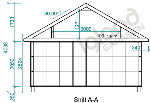
Snitt A-A
