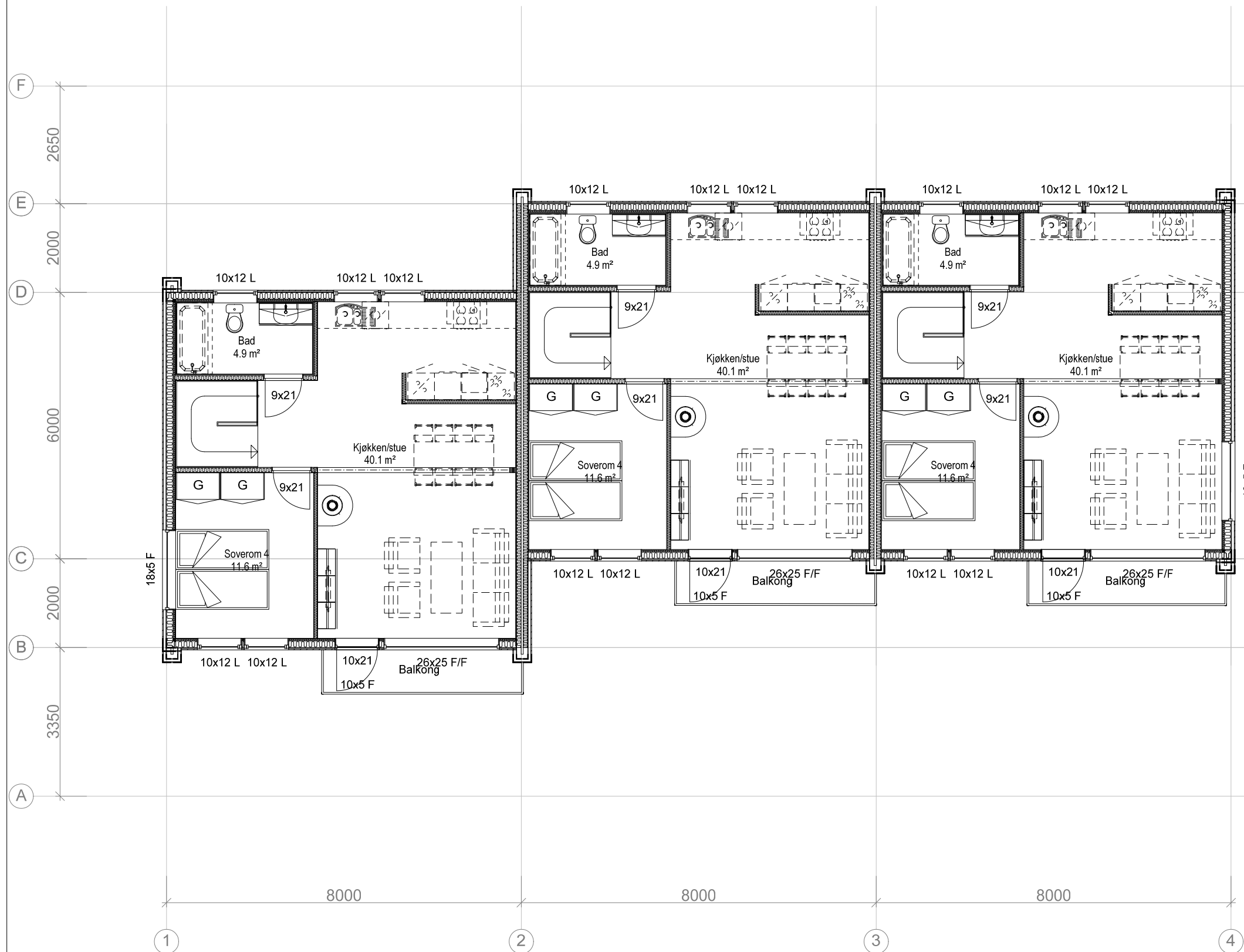
BOLIG 41 Plan 2. etasje BRA 58,1 m2
