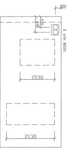
Plan kjeller
