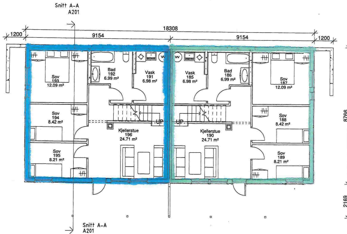
Plan 01 1 : 100
