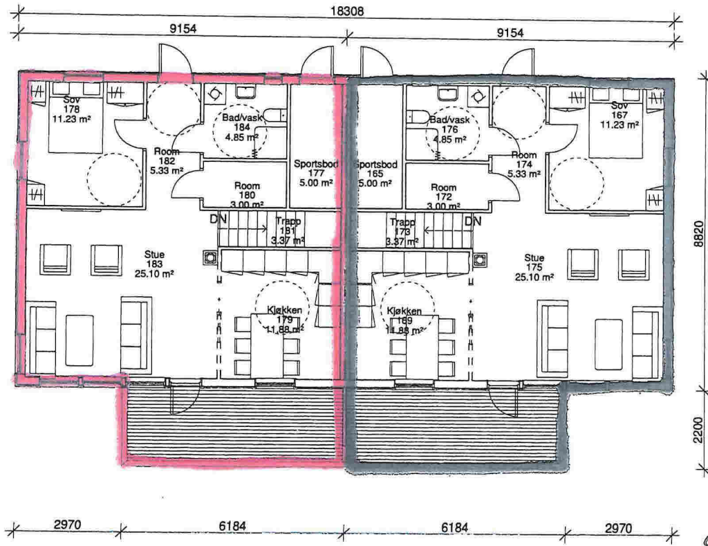
Plan 02 1 : 100
