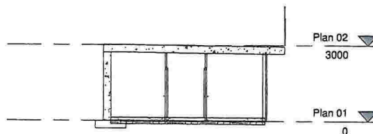
Snitt B-B 1 : 100
