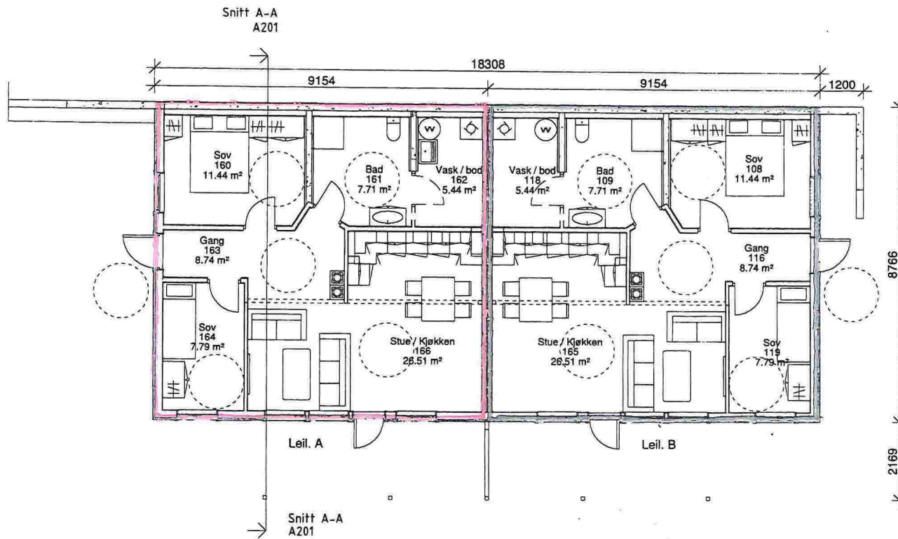
Plan 01 1 : 100
