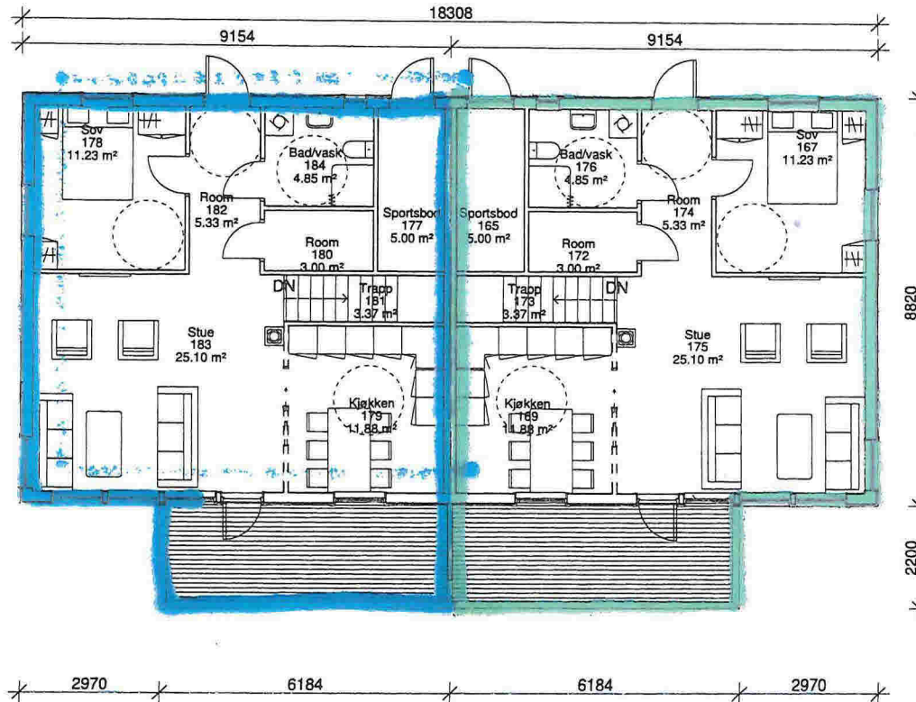
Plan 02 1 : 100
