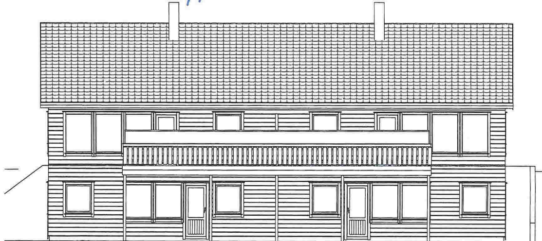
Fasade Øst 1 : 100
