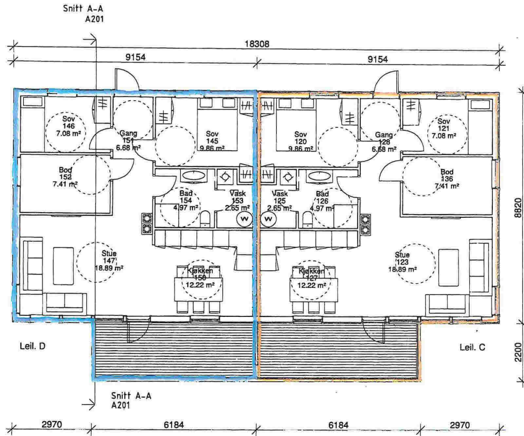
Plan 02 1 : 100
