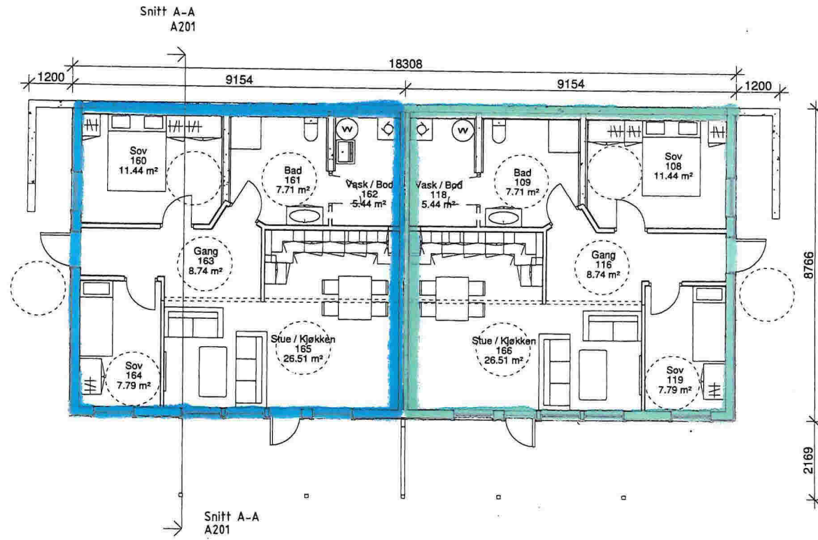
Plan 01 1 : 100
