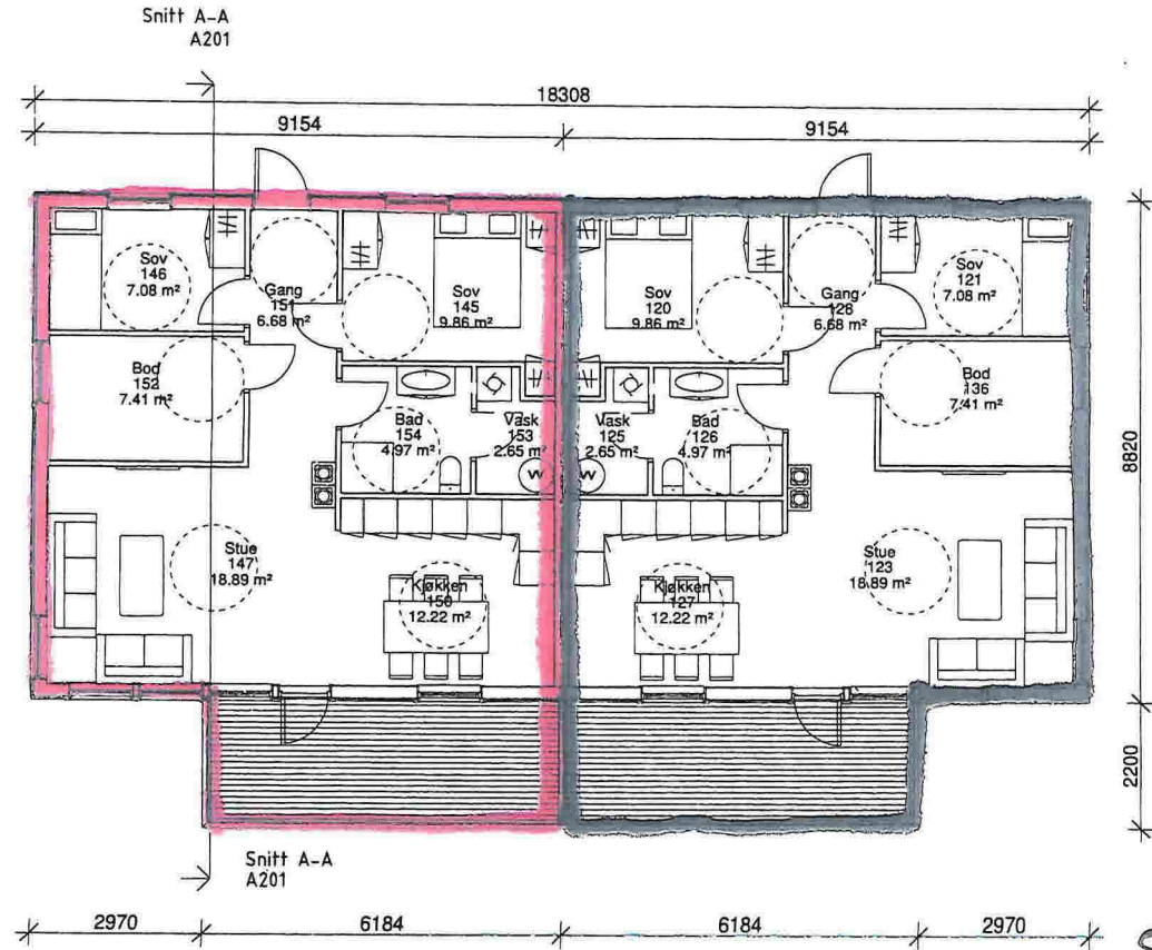
Plan 02 1 : 100
