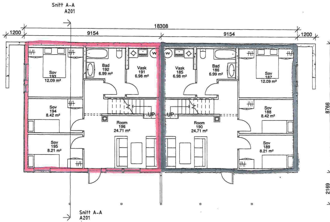
Plan 01 1 : 100
