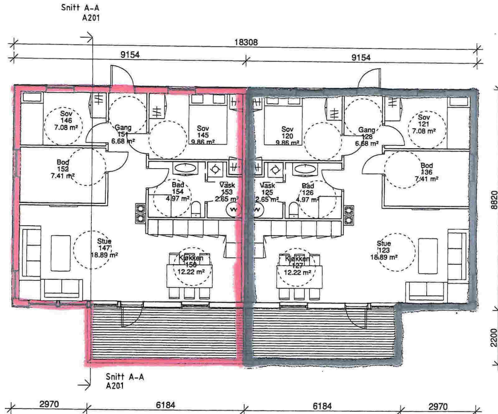
Plan 02 1 : 100
