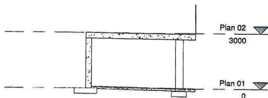
Snitt A-A 1 : 100
