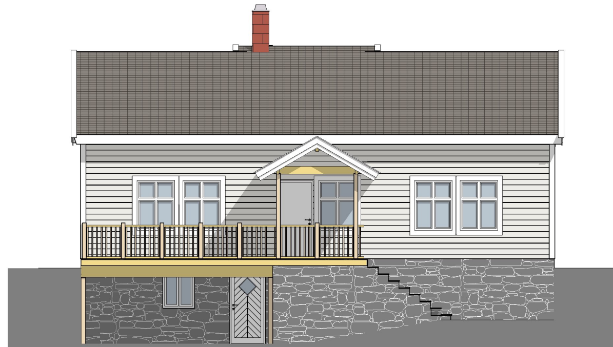
1:100 Fasade Sør
