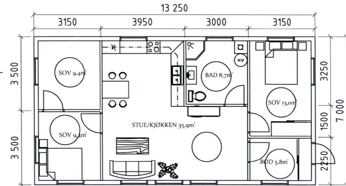
PLAN 1 ETASJE
