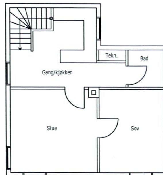
PLAN 2 ETASJE
