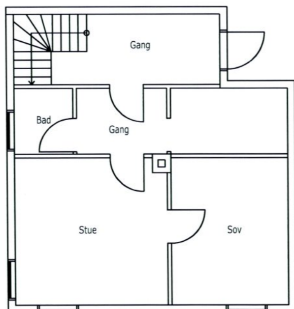
PLAN 1 ETASJE
