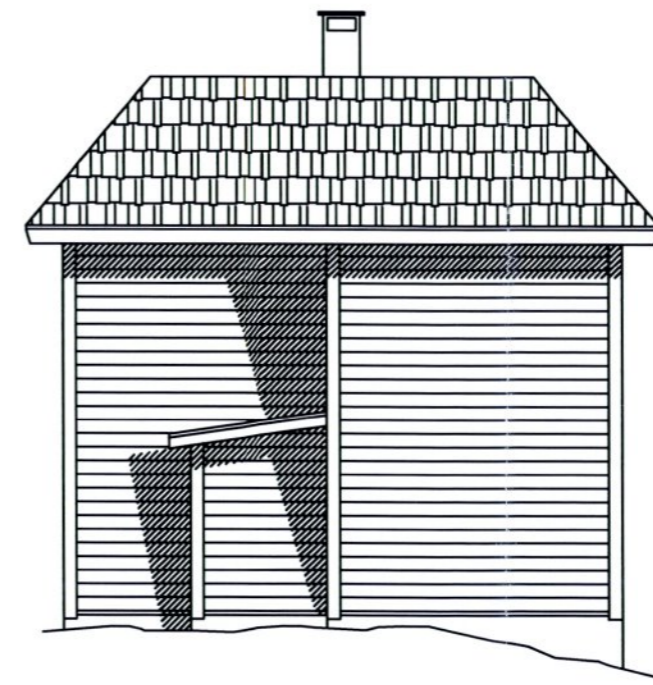
FASADE ØST
