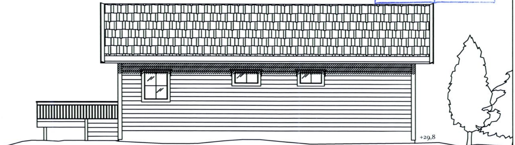
FASADE ØST
