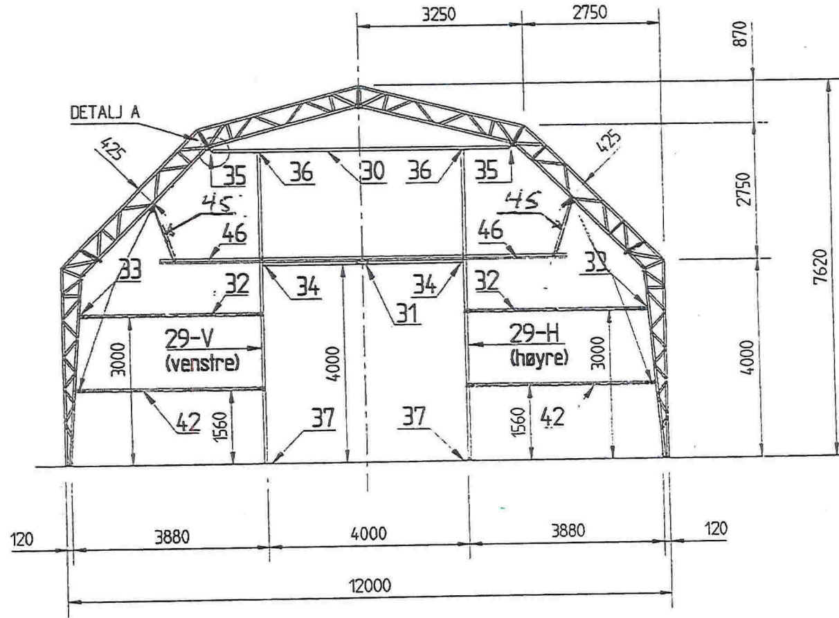
OPPRISS GAVLFORGITRING 1:100
