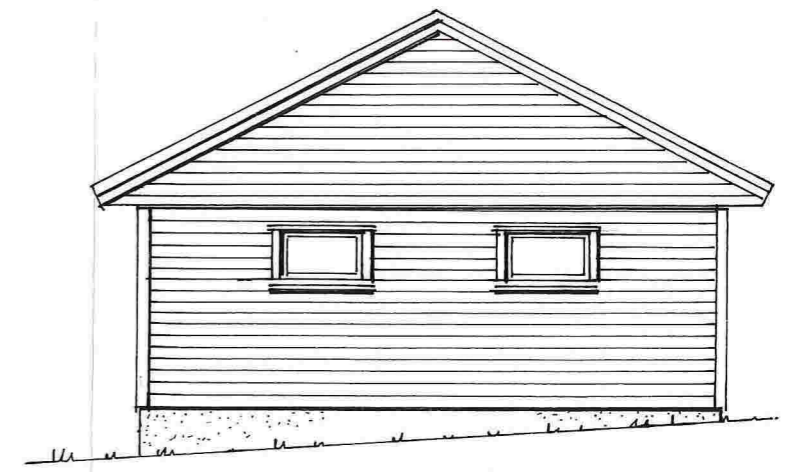
Fasade mot SYD-ØST
