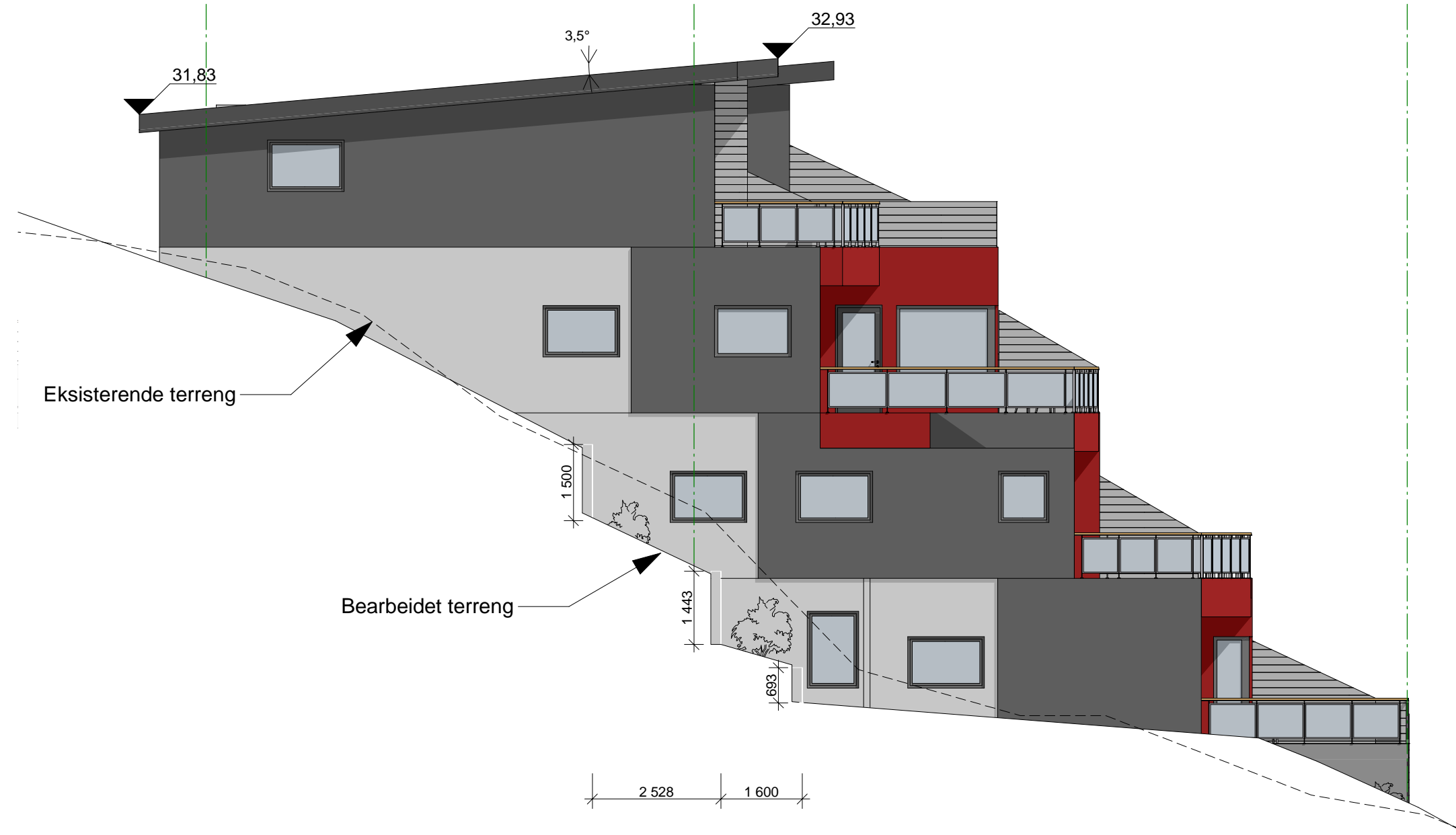
1:100 Fasade Nord
