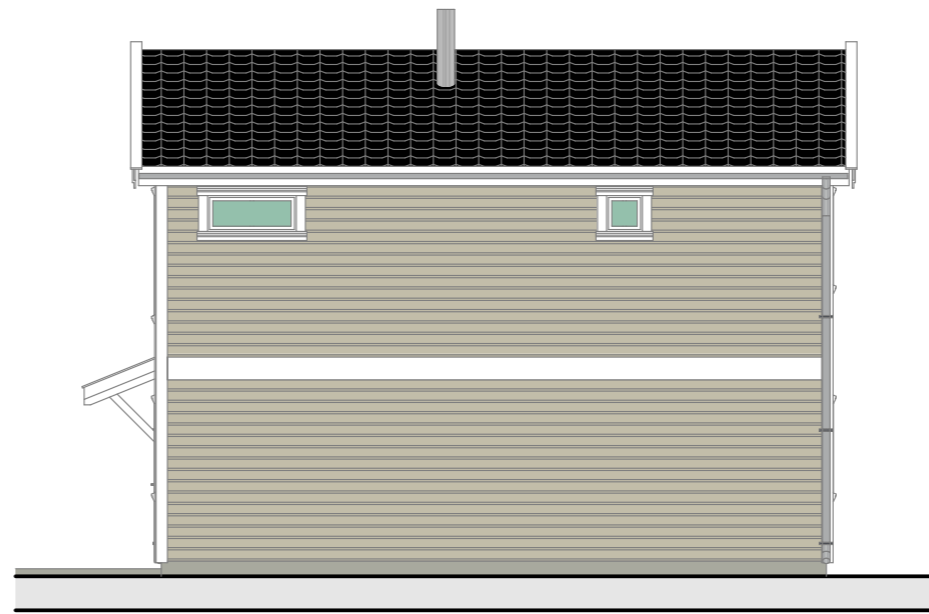
Øst Øst 1:100
