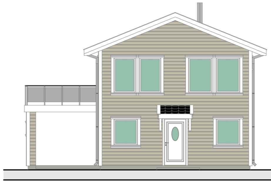
Syd Syd 1:100
