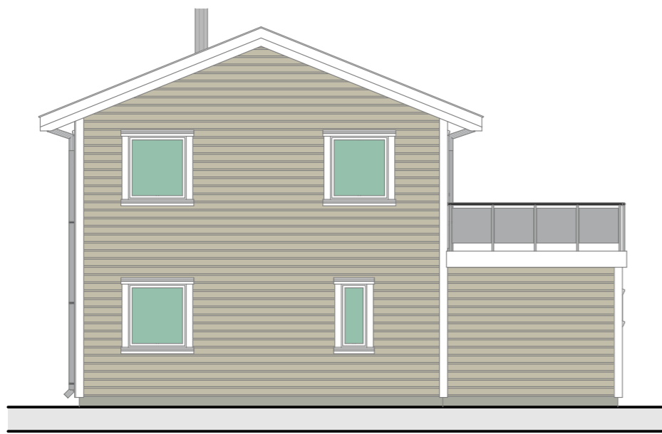
Nord Nord 1:100
