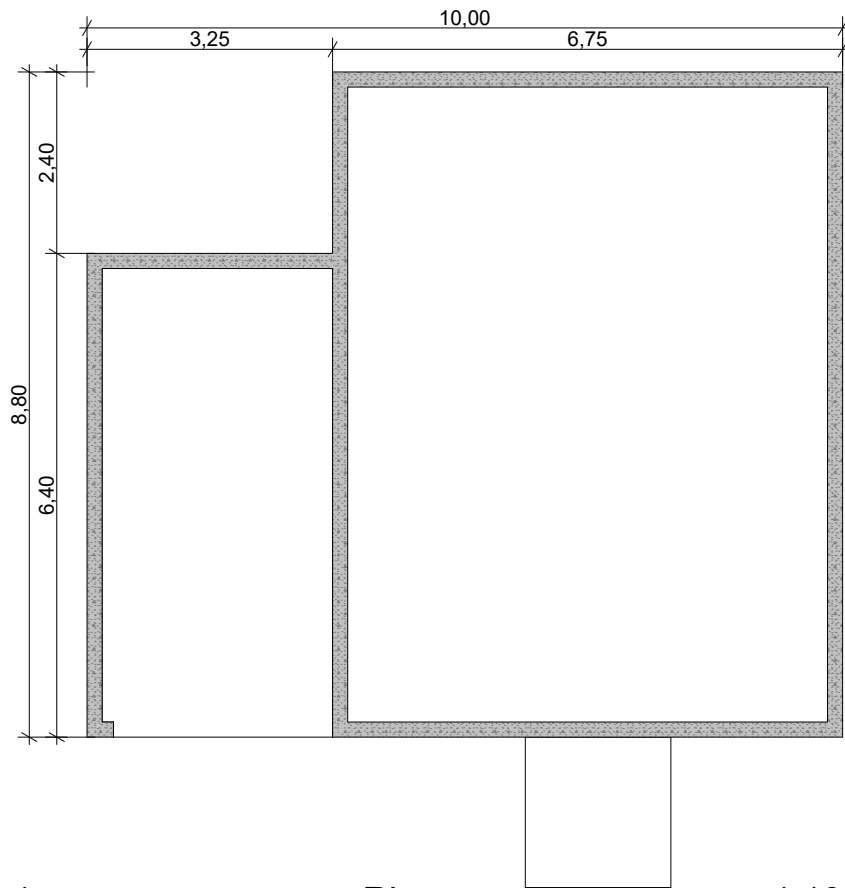
-1. Ringmur 1:100 0.
