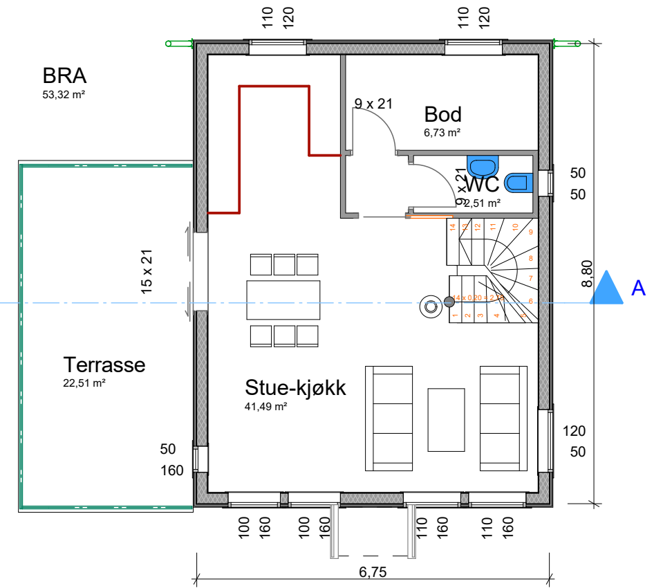
2 etasje 1:100
