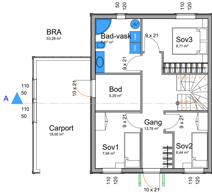
1 etasje 1:100 1.
