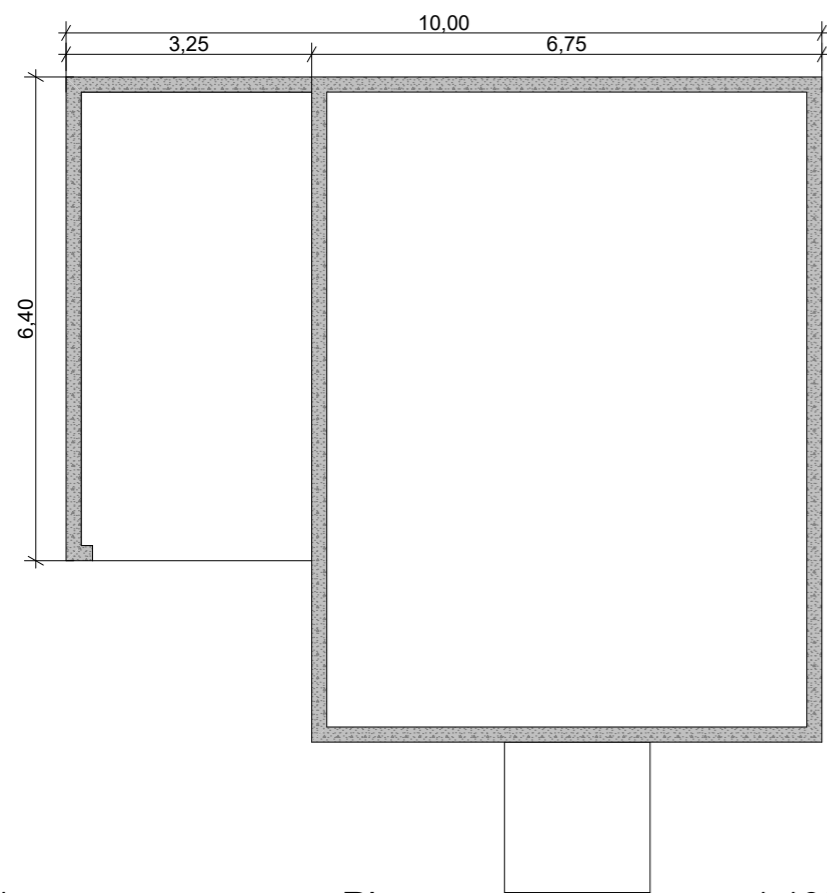
-1. Ringmur 1:100 0.
