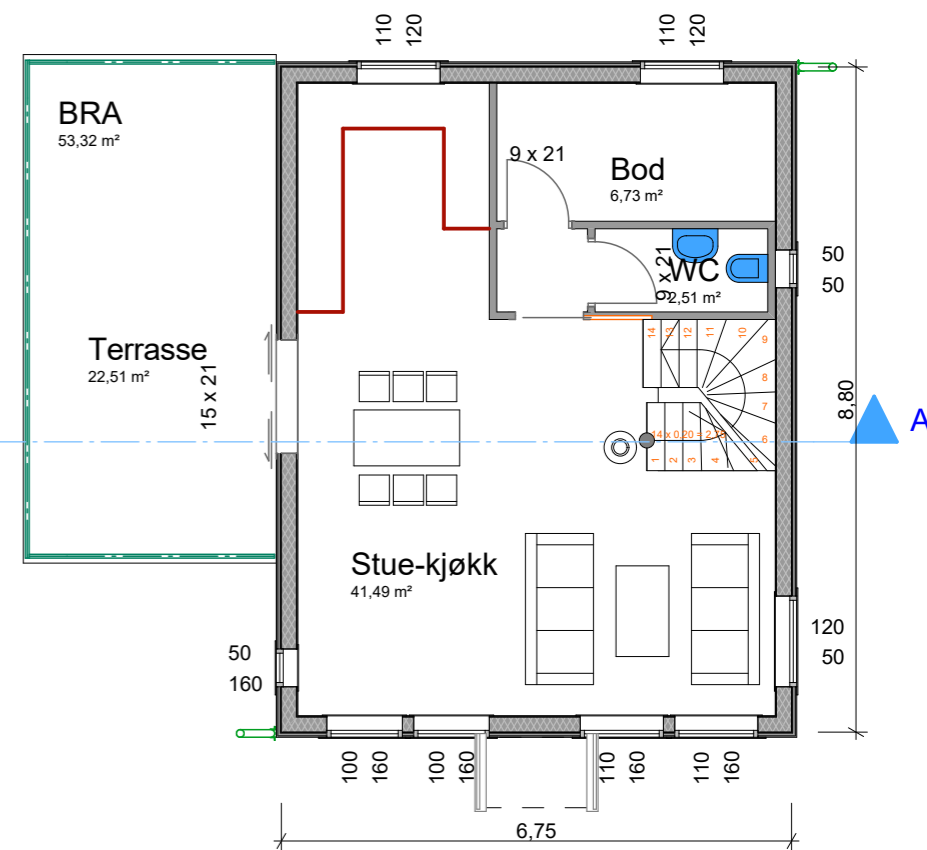
2 etasje 1:100
