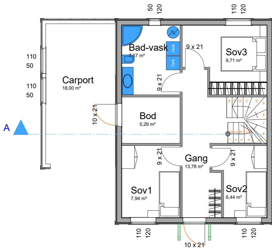
1 etasje 1:100 1.
