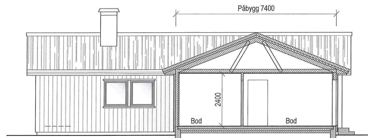
SNITT B
