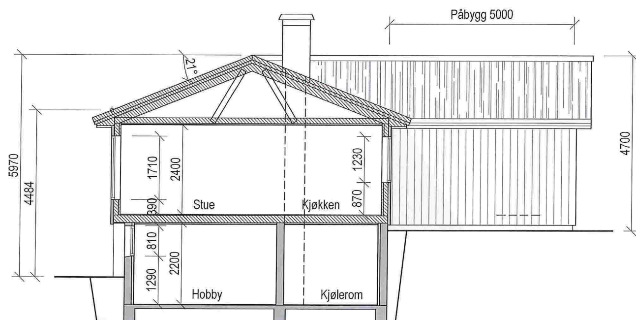
SNITT A
