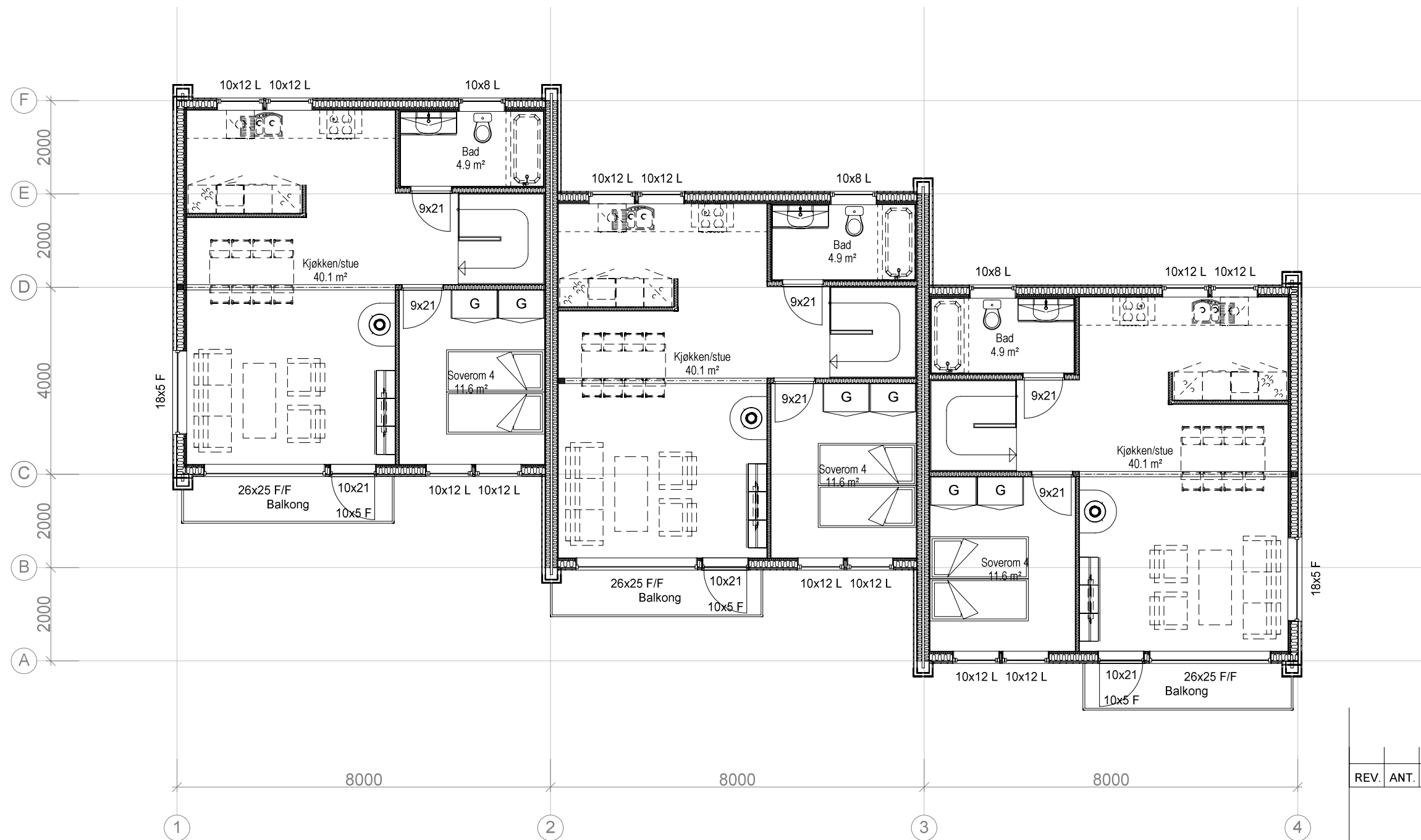
BOLIG 38 Plan 2. etasje BRA 58,1 m2
