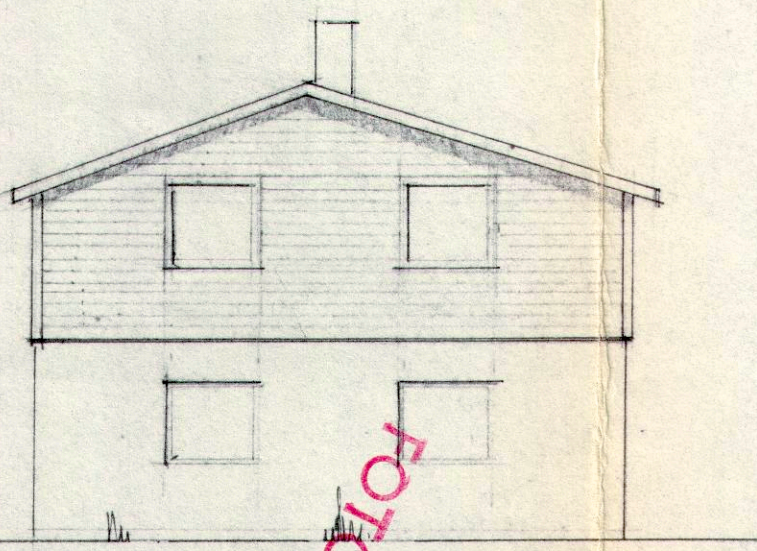
MOT NORD
