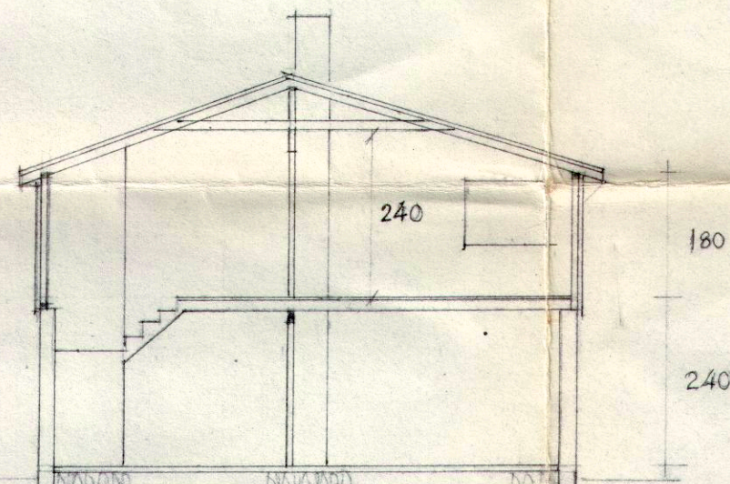
SNITT TILBYGG
