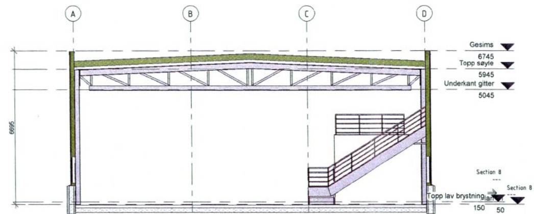
Snitt A-A 1 : 75
