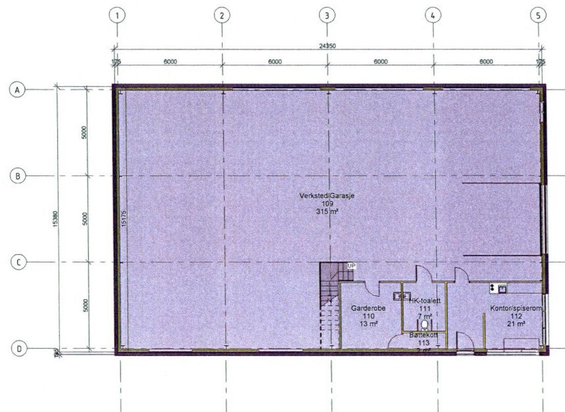
Plan 01 1 : 100
