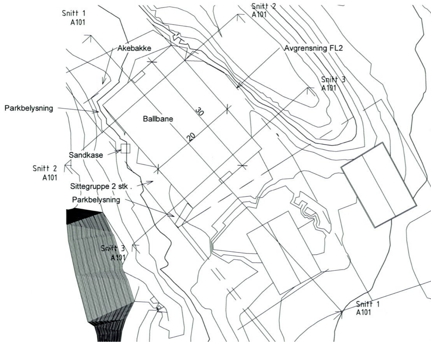
Situasjon FL2 1 : 500
