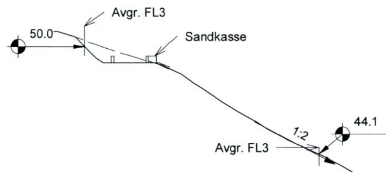
Snitt A-A 1 : 200
