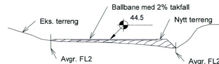
Snitt 3 1 : 500
