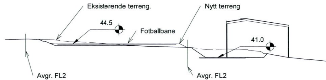
Snitt 1 1 : 500
