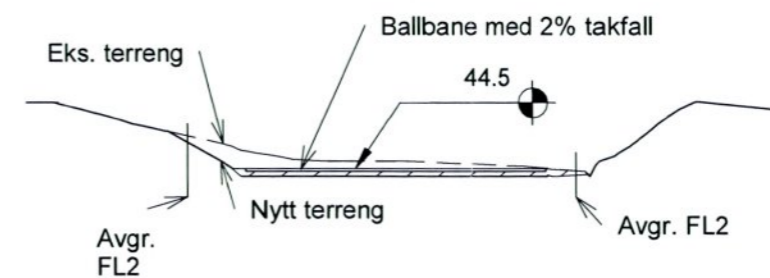
Snitt 2 1 : 500
