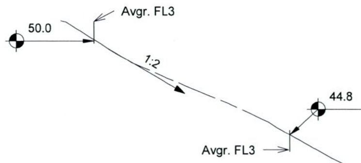
Snitt B-B 1 : 200
