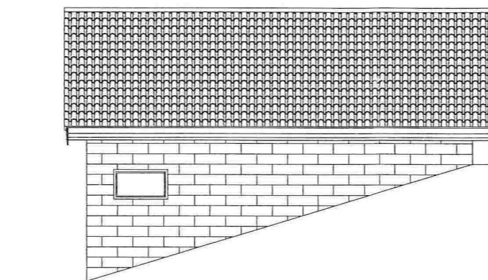
Fasade mot:Øst
