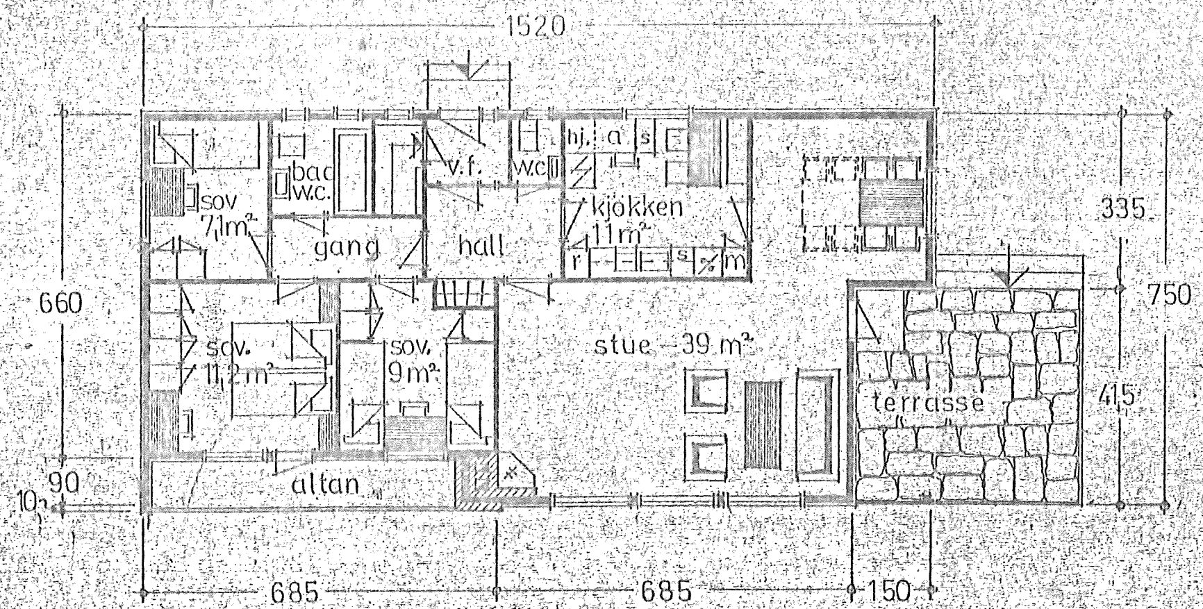
PLAN AV 1. ETG.
