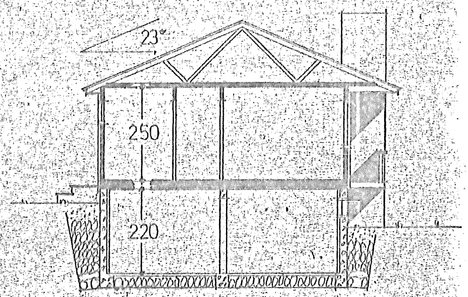
SNITT.
