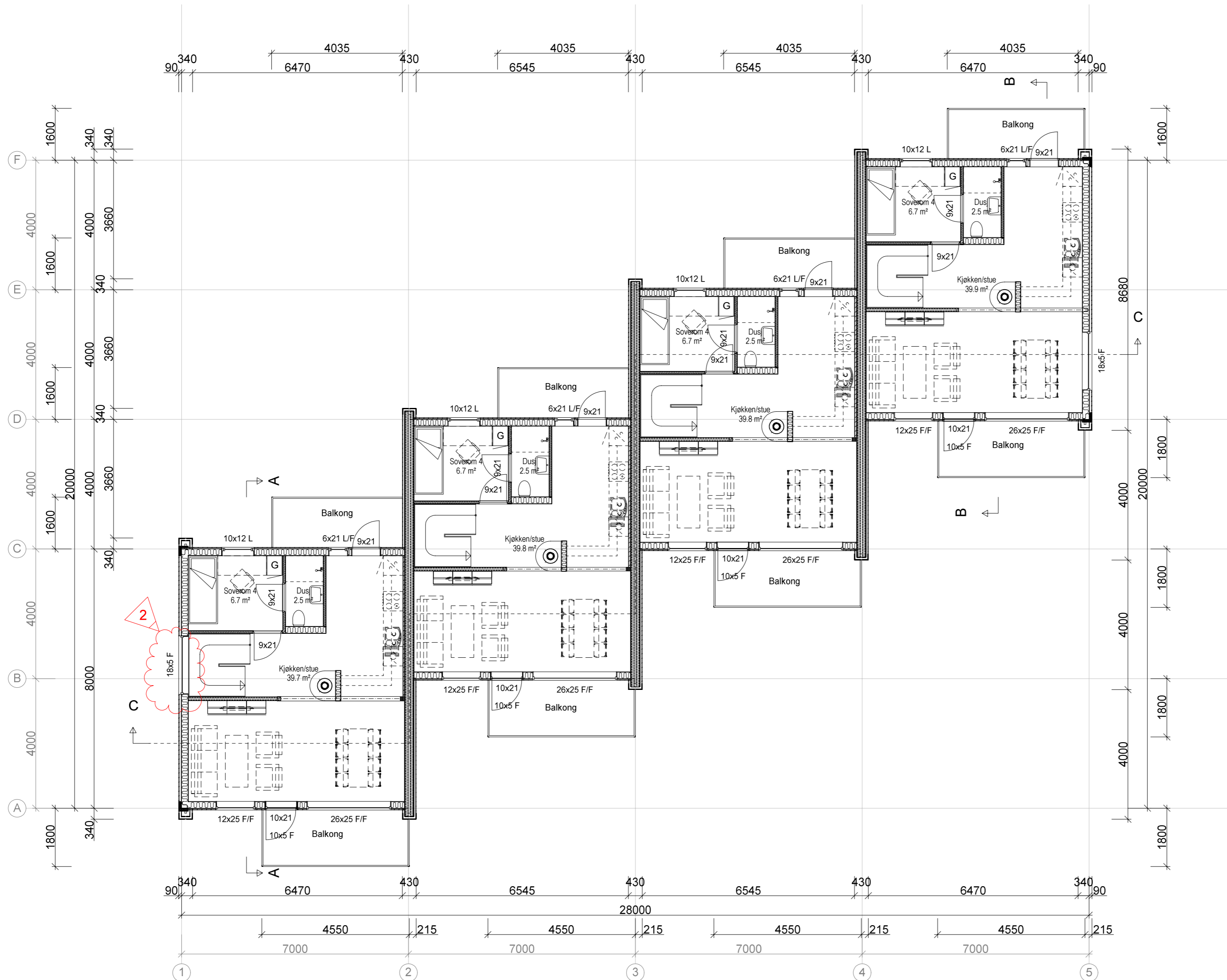
BOLIG 26 Plan 2. etasje BRA 50,2 m 2
