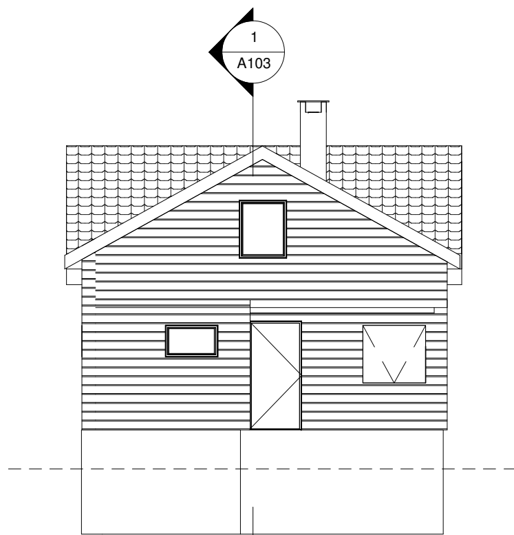
3 sør-øst 1 : 100
