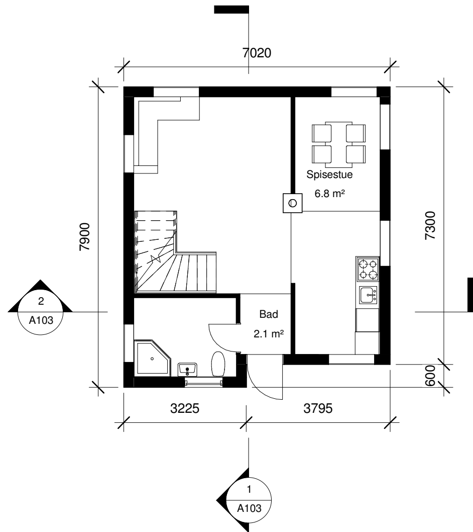
1 1 - 1. etasje 1 : 100
