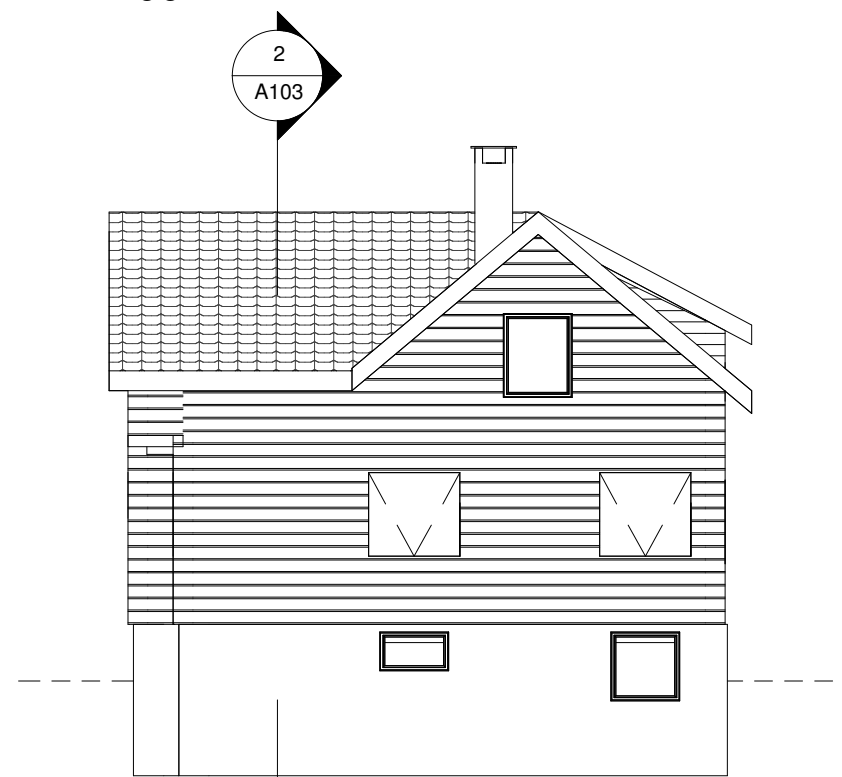
4 sør-vest 1 : 100
