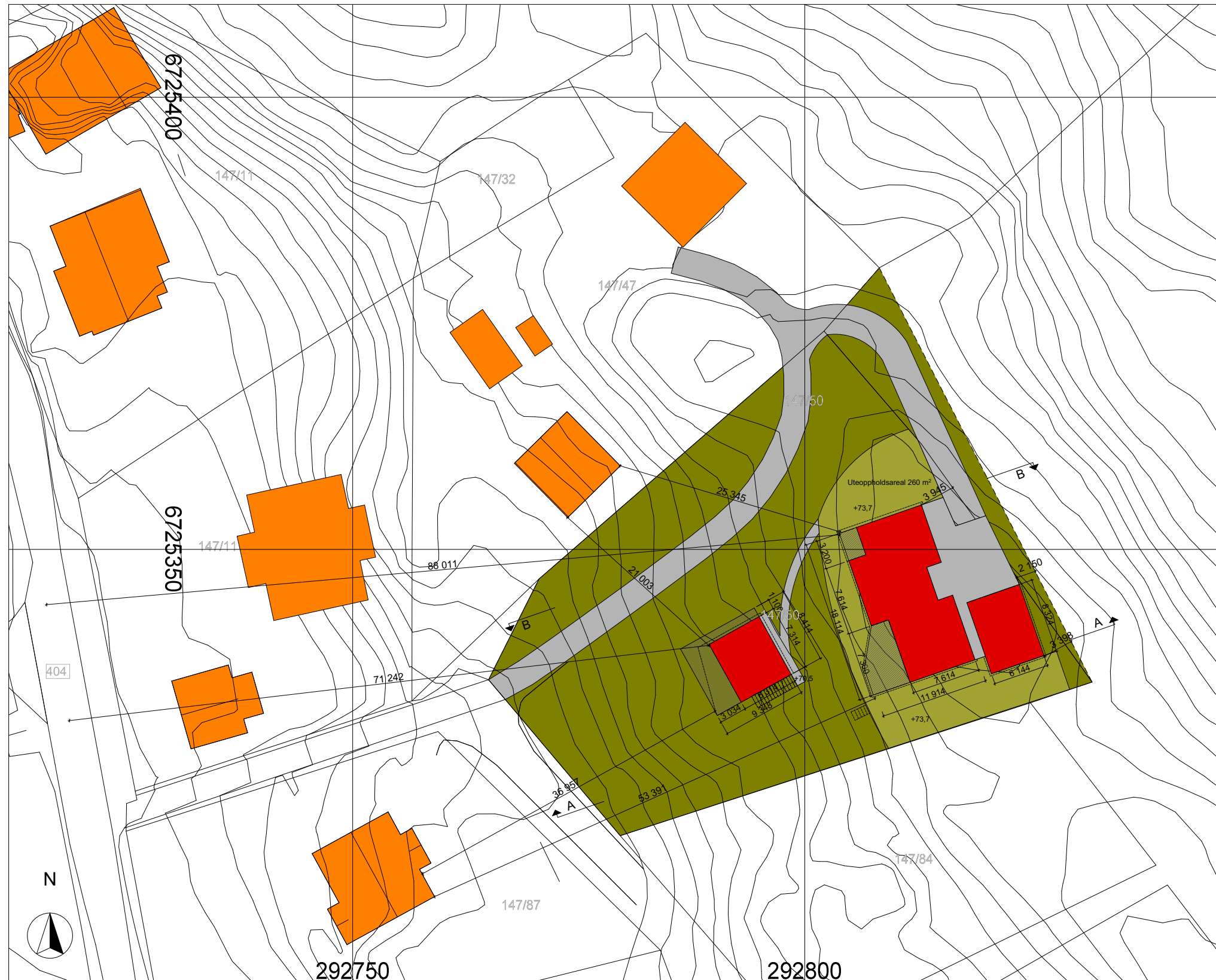
1:500 Situasjonsplan
