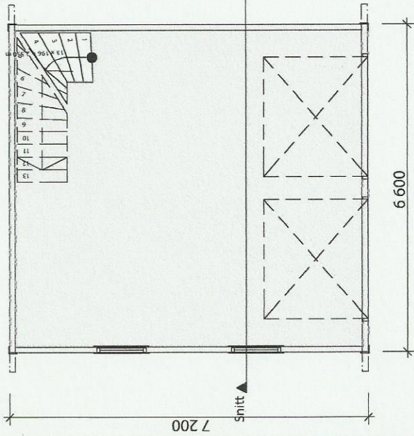
Plan 1 etasje 1:100
