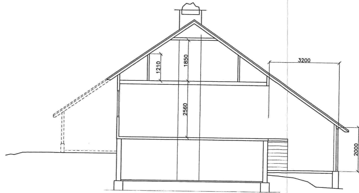
SNITT B-B
