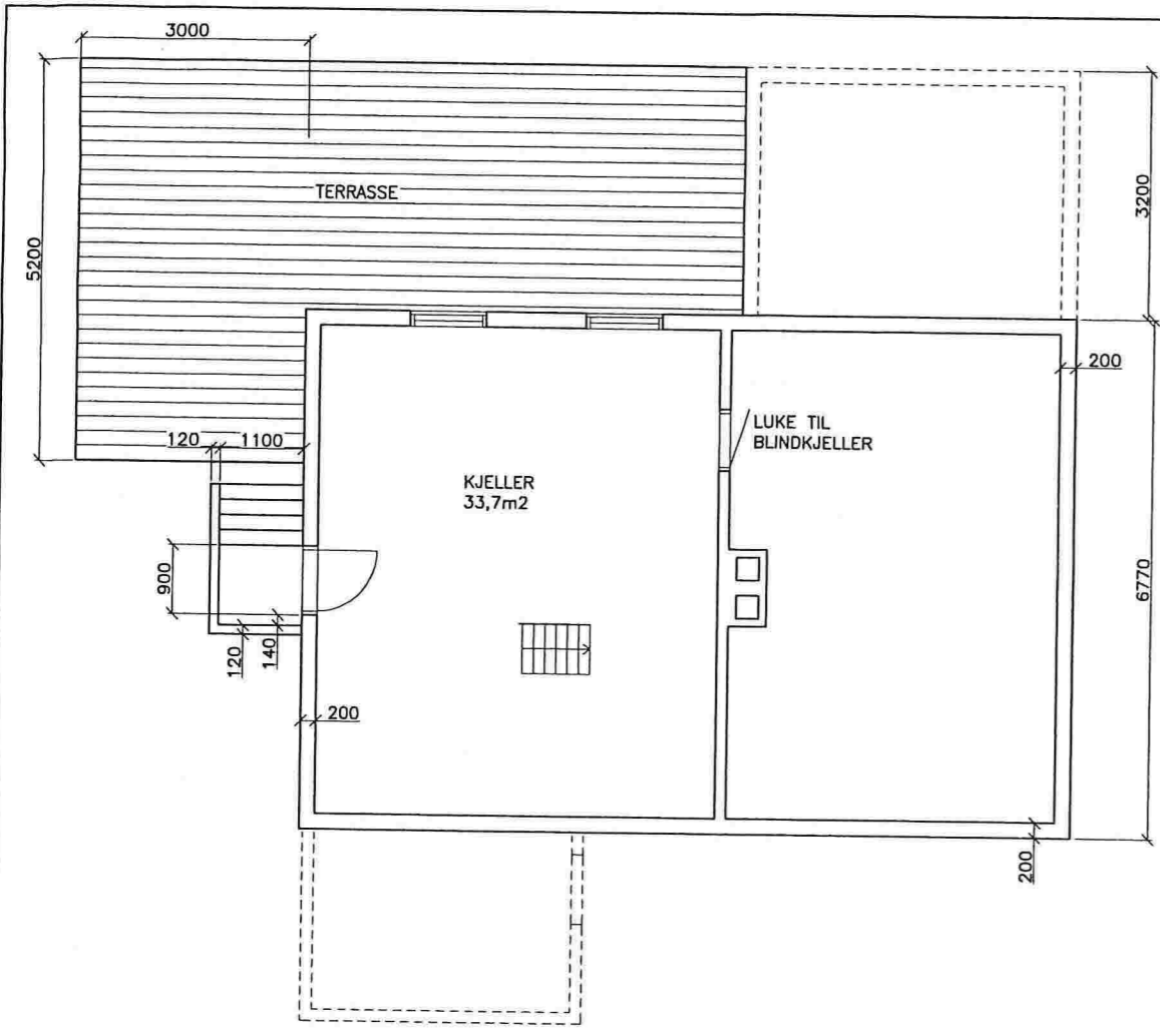
PLAN KJELLER
