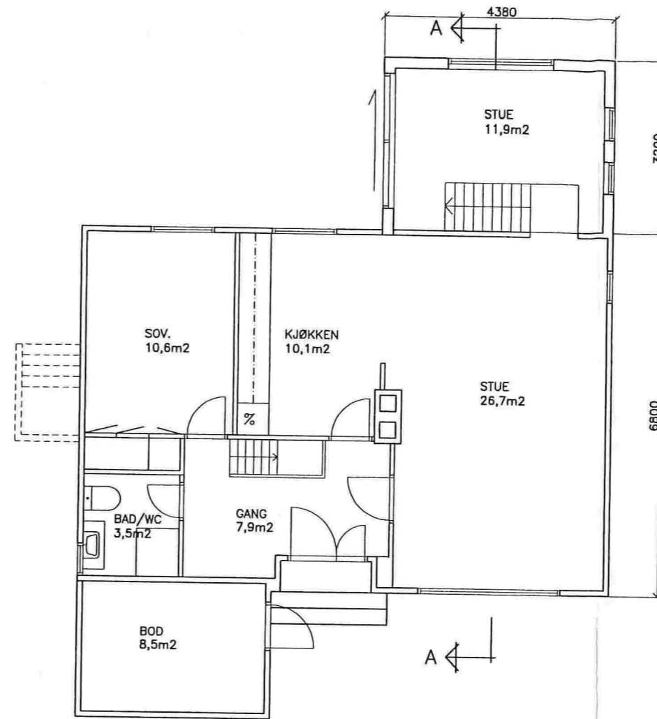
PLAN 1.ETASJE
