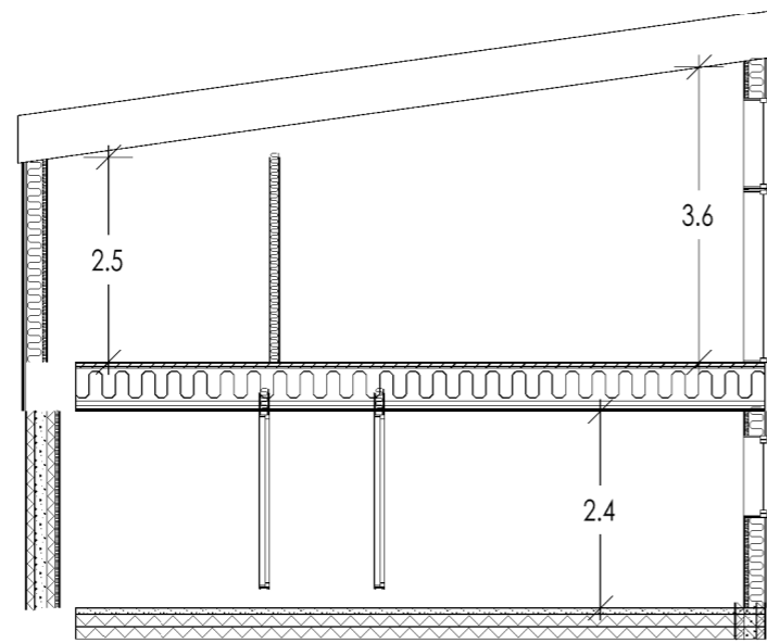
Snitt B-B
