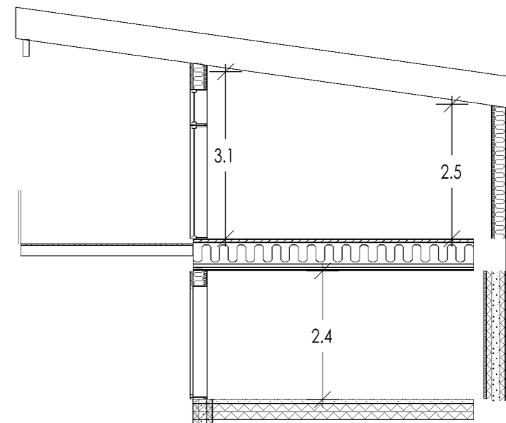
Snitt A-A
