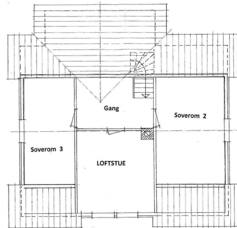
Plan av LOFTSETASJE
