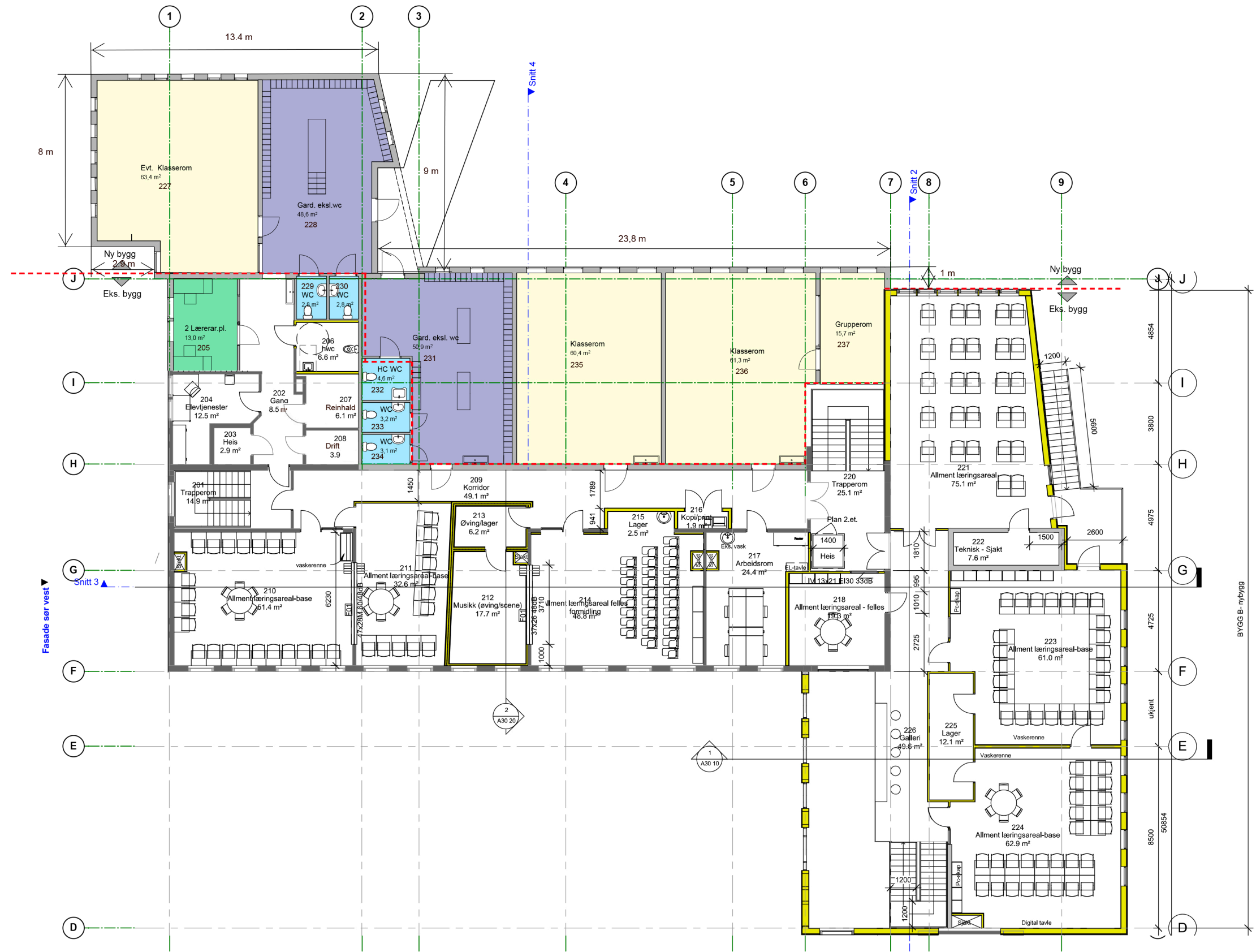
1:200 2.etg
