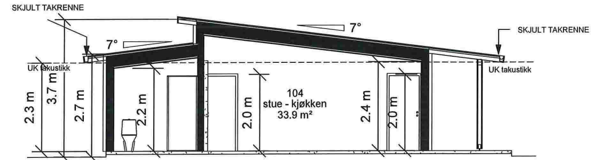
SNITT A-A
