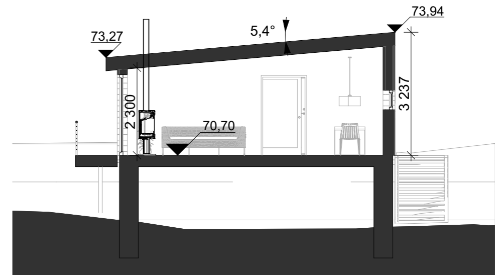
1:100 Snitt A
