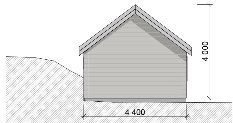
fasade Vest
