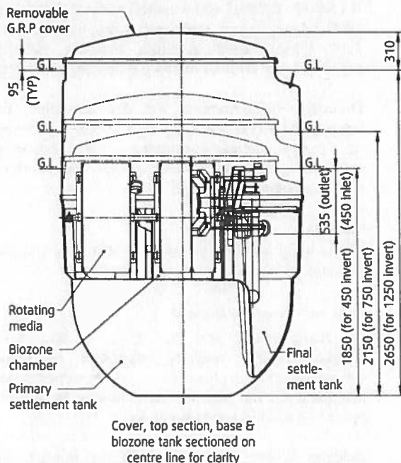
Figur 1. Skisse av rensanlegget sett fra siden (Biodisc BA).
