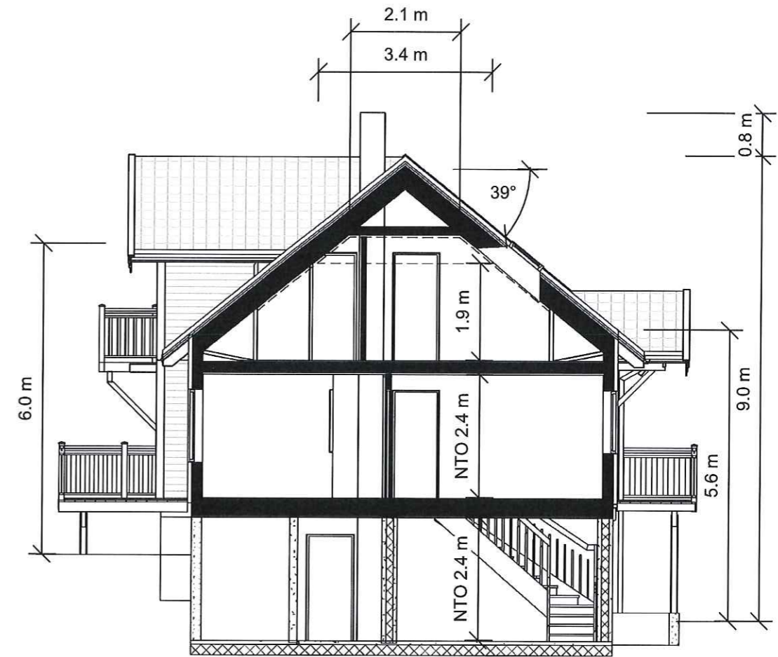
SNITT A-A
