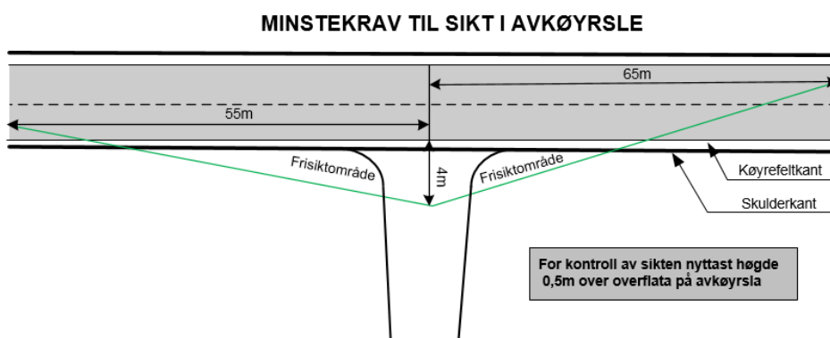
Fig. Prinsippskisse minstekrav til sikt
