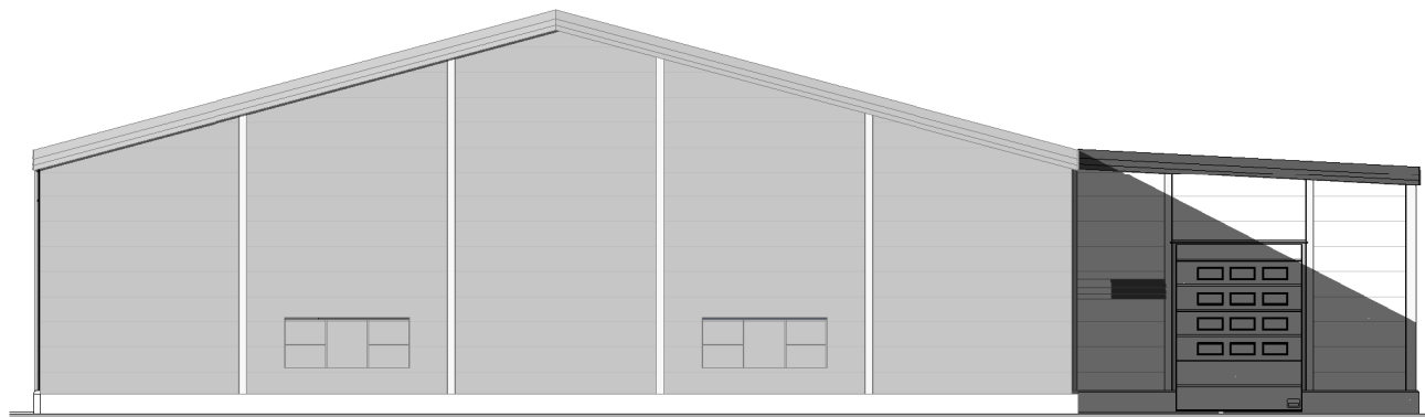
2 Sør-vest 1 : 200
