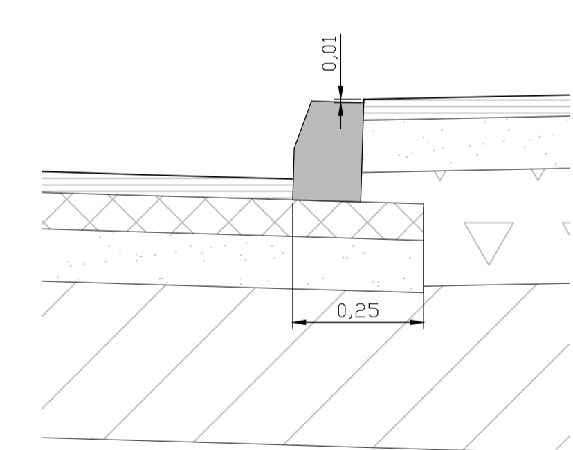
DETALJ FORTAUSKANT M=1:10
