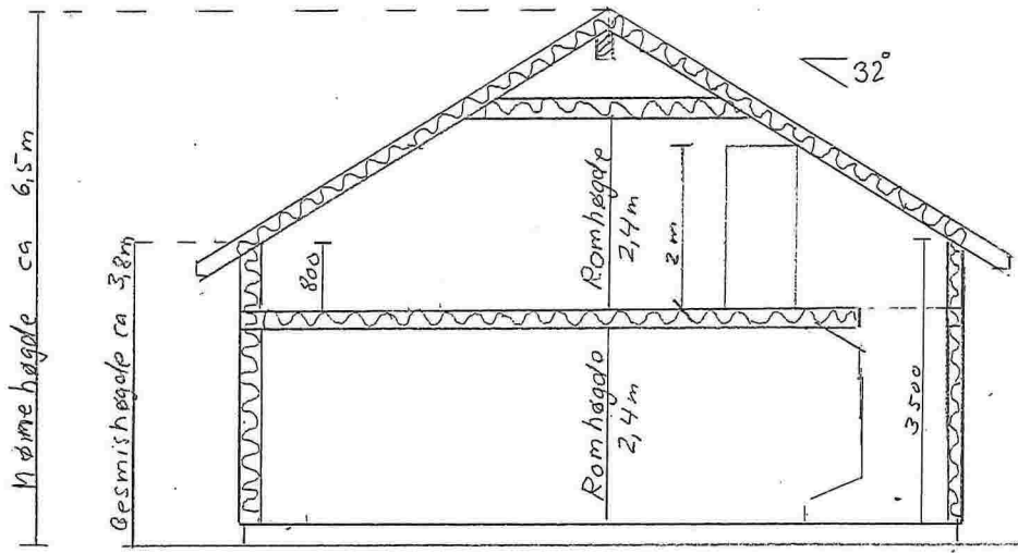
SNITT B-B
