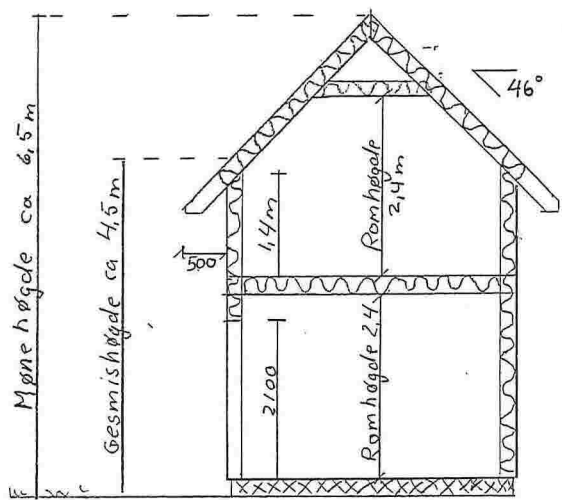
SNITT A-A
