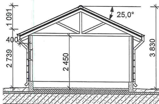
Snitt 1:100
