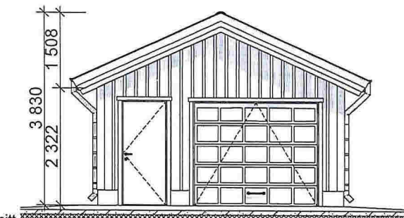
Fasade 1 1:100
