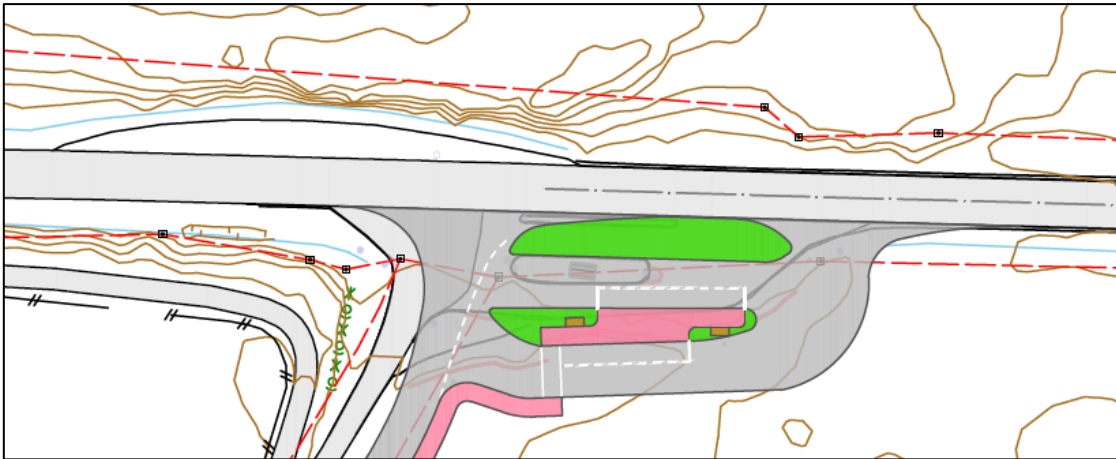
Eksempel på utforming på snuplass for bussar, Utsnitt frå teknisk vegplan, Statens vegvesen
