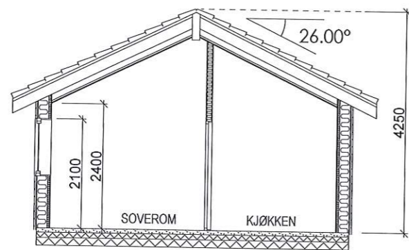
SNITT A-A
