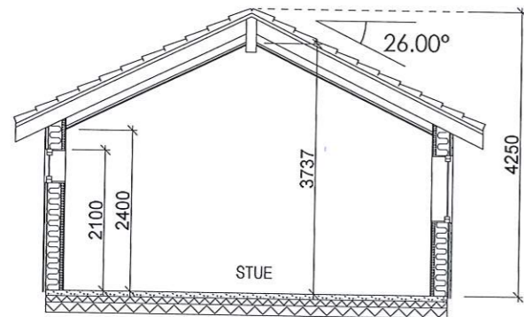
SNITT B-B
