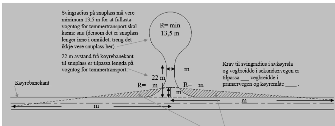
Fig: Døme prinsippskisse tømmeravkøyrsløse med snuplass.
