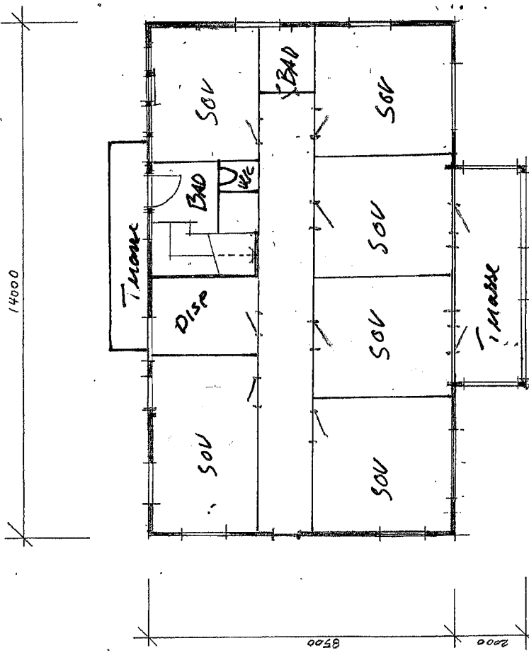
PLAN 1. ET.
