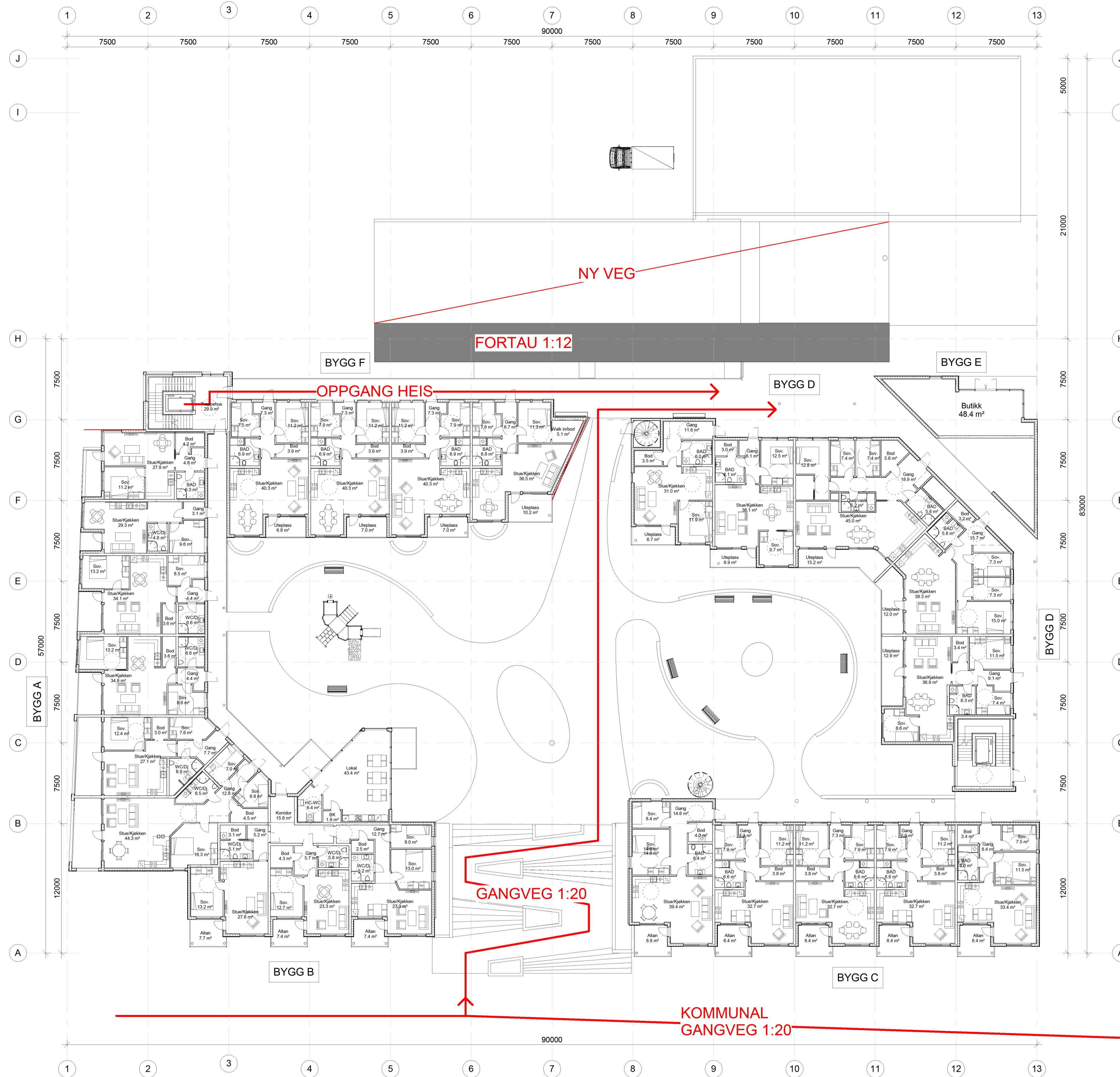
1 Plan 02 - Gangveier 1 : 200
