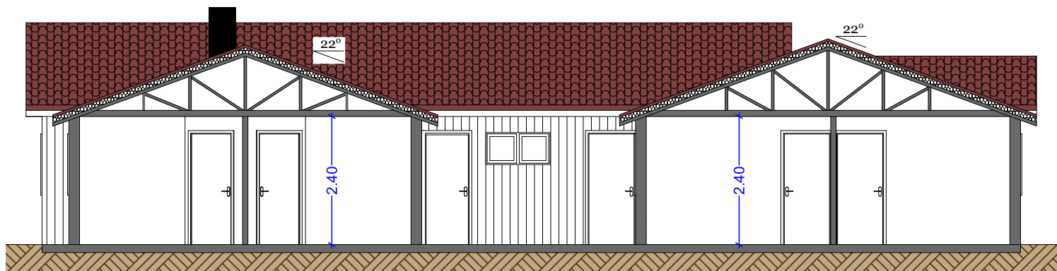
Snitt A-A
